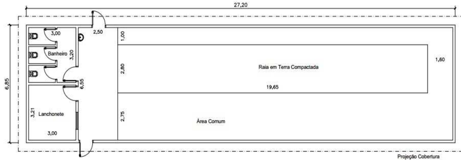
PLANTA BAIXA ESCALA: 1:100
