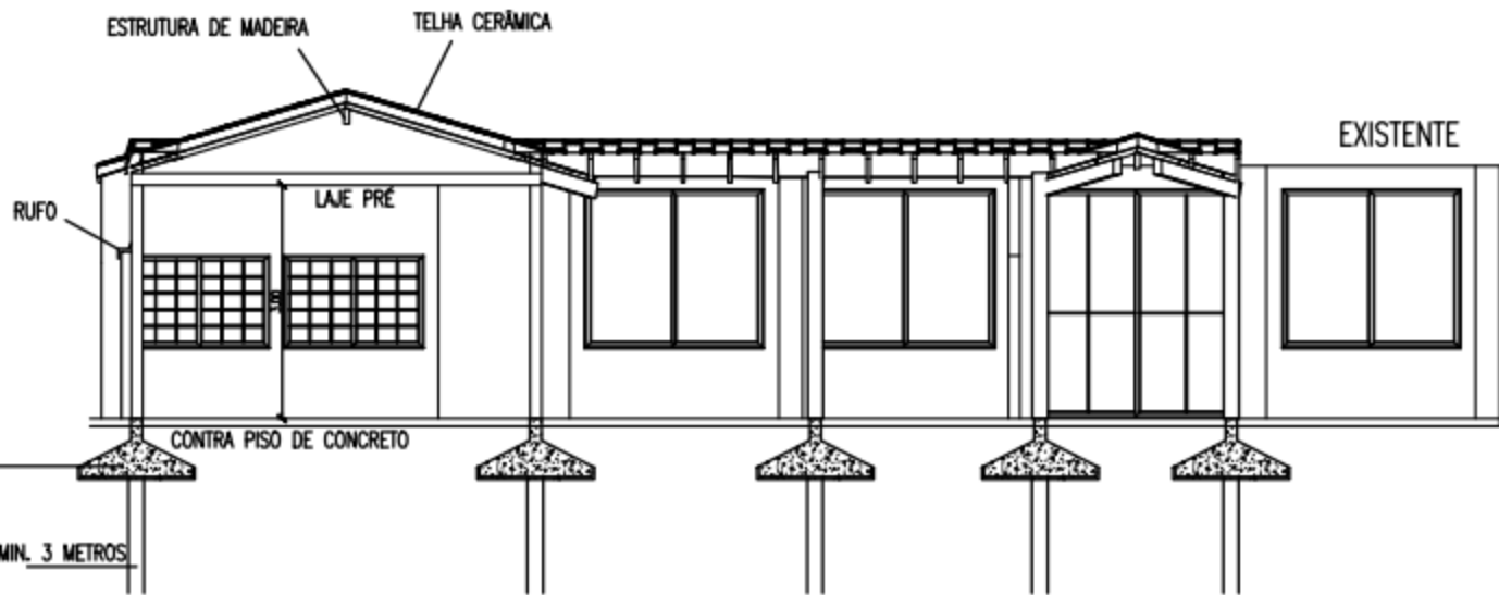
Corte 2-2
