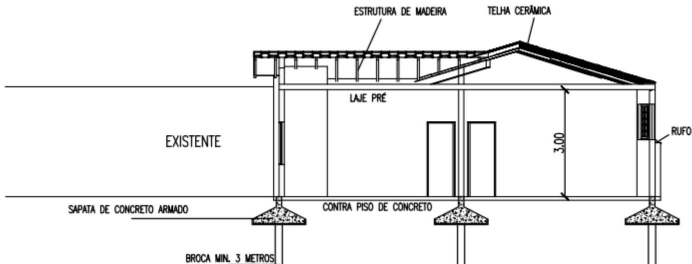
Corte 1-1
