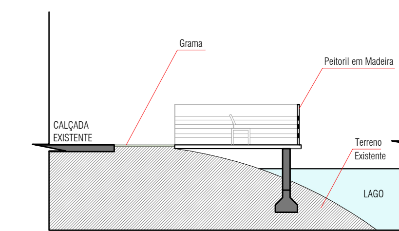
DETALHAMENTO DECK INDICAÇÕES ESCALA 1: 100
