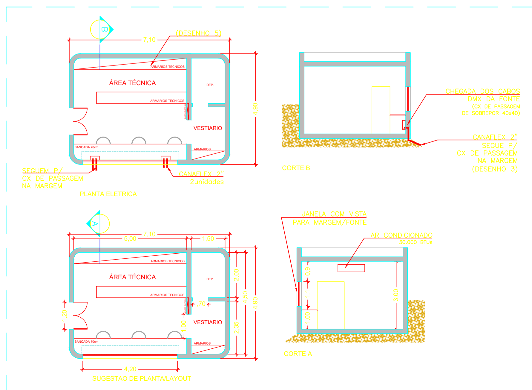
2 ABRIGO - SALA DE CONTROLE ESCALA 1:100
